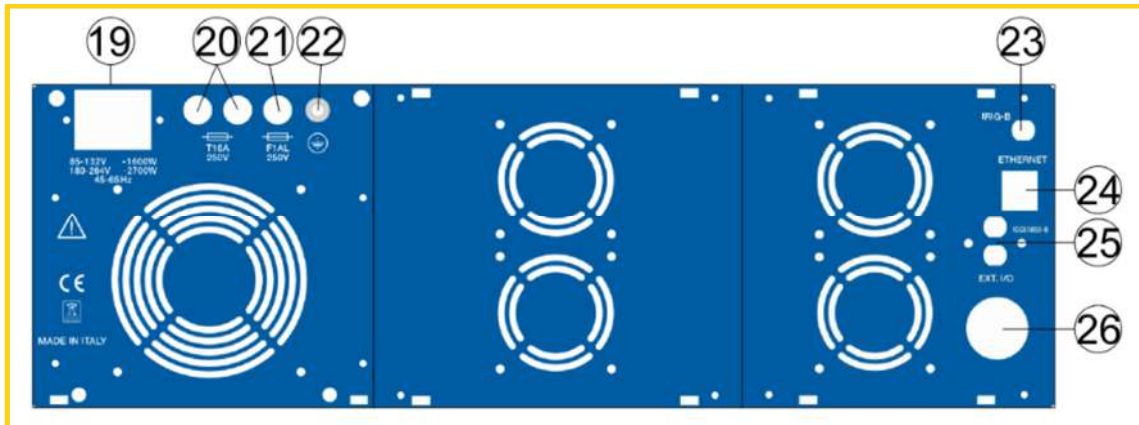
Figura 2 – Pannello posteriore
